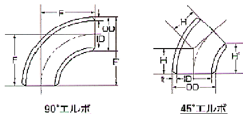
90°エルボ
